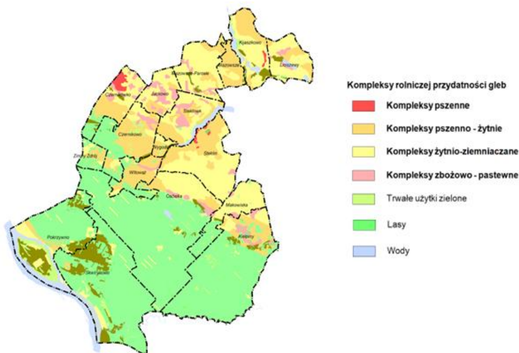
Rysunek 5. Kompleksy rolniczej przydatności gleb w gminie Czernikowo
