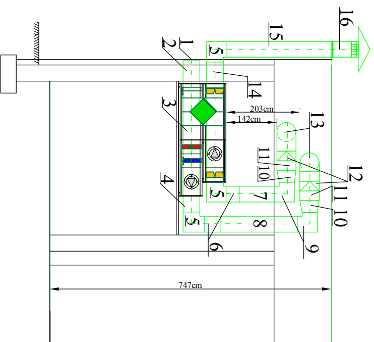
PRZEKRÓJ PIONOWY A-A
